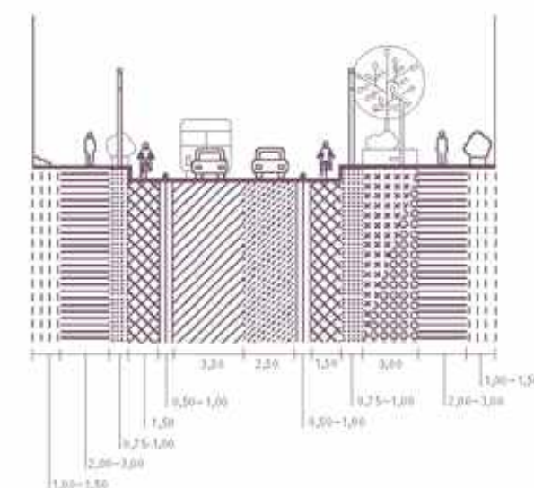
Схема. 57. Функциональное зонирование улицы типа 7Ц. Вариант Б
