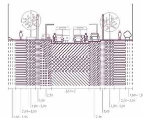
Схема. 56. Функциональное зонирование улицы типа 7Ц. Вариант А
