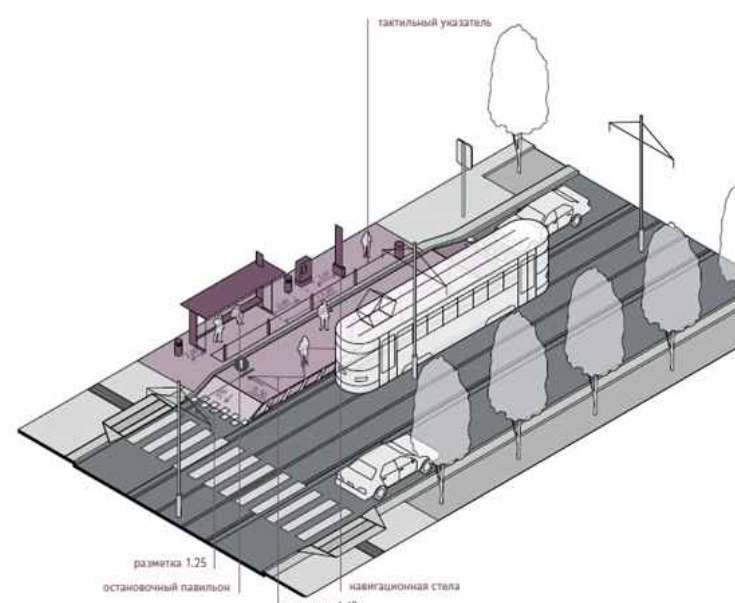
Схема 110. Остановочный пункт трамвая пражского типа
